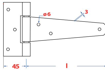
T-Hinge
