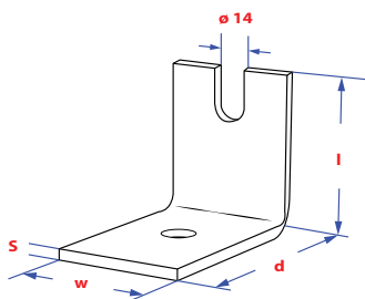
Angled lug
